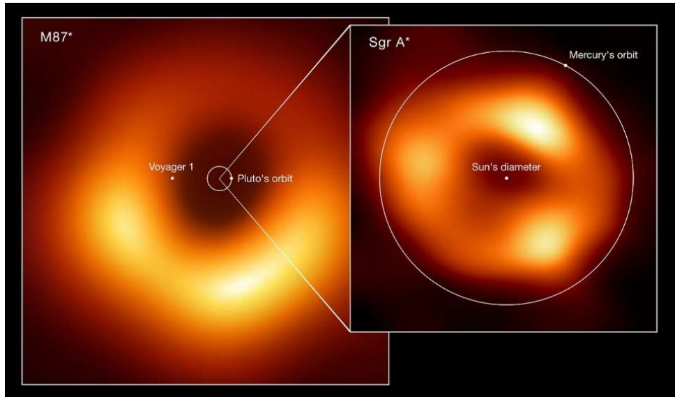
Bild 3 Größenvergleich der Schwarzen Löcher in M87 und der Milchstraße 8
