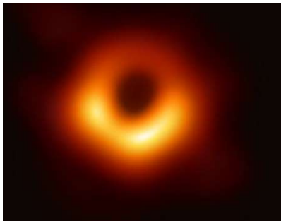
Bild 1 Schwarzes Loch in der Galaxie Messier 87 4 (Foto: EHT Collaboration)
