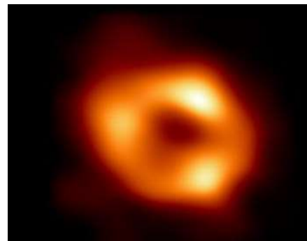
Bild 2 Schwarzes Loch im Zentrum der Milchstraße 6
