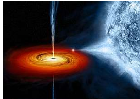
Bild 1 Künstlerische Darstellung von Cygnus X-1 3
